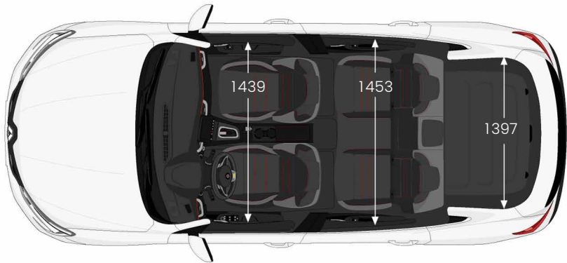
Dimensions (mm).
